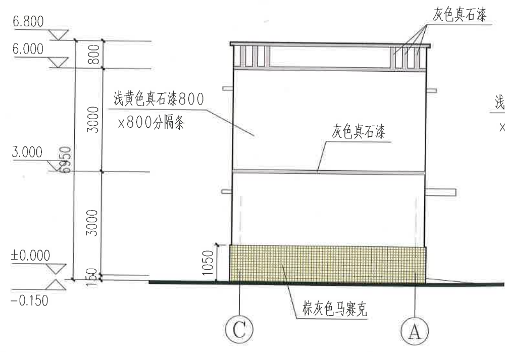
C—A立面图 1:100
