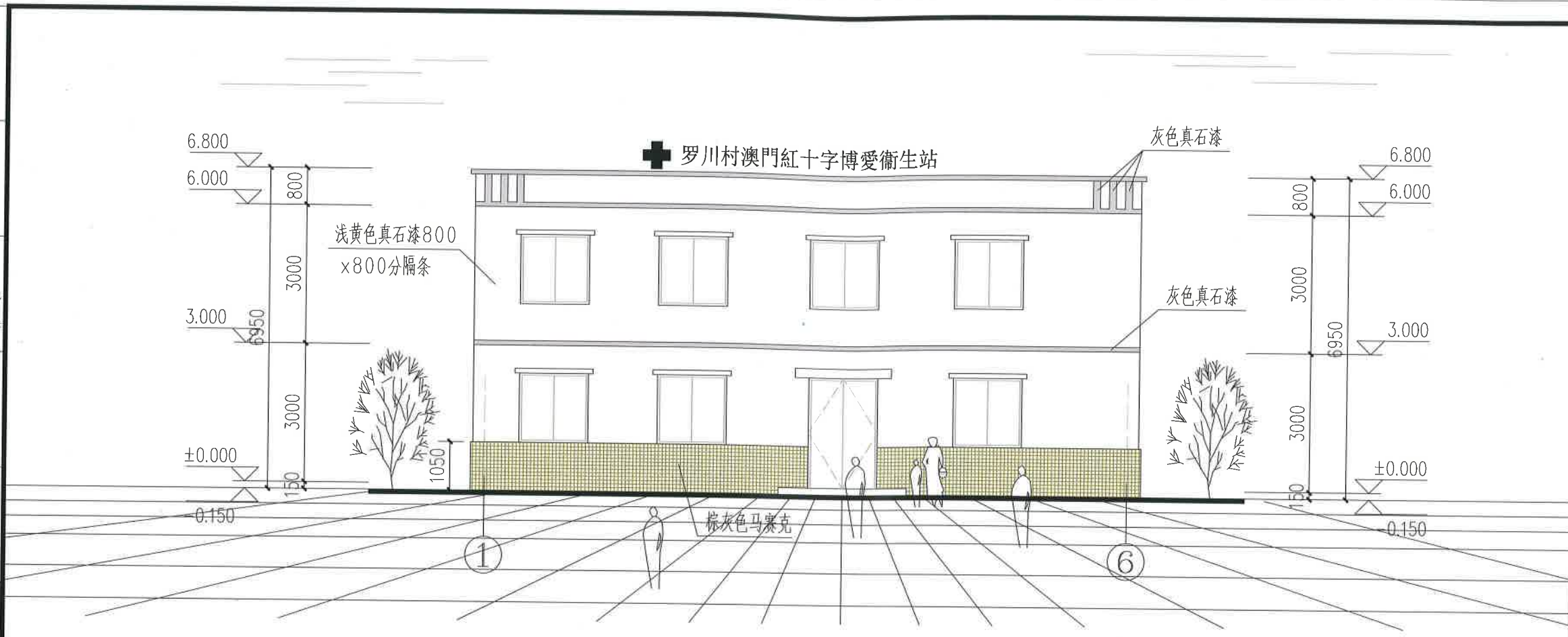
①—⑥立面图 1:100
