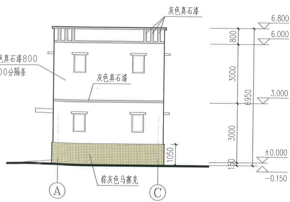
A—C立面图 1:100
