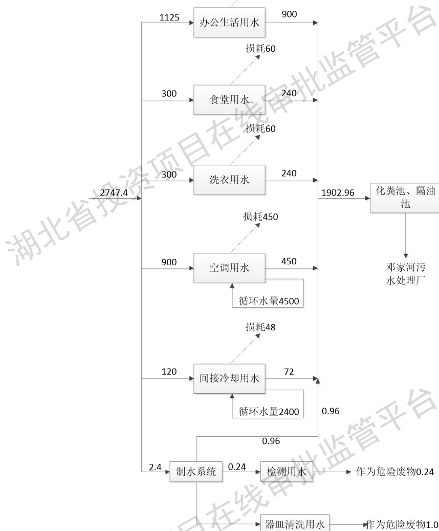
图4-1 拟建项目水平衡图 单位：m³/a
