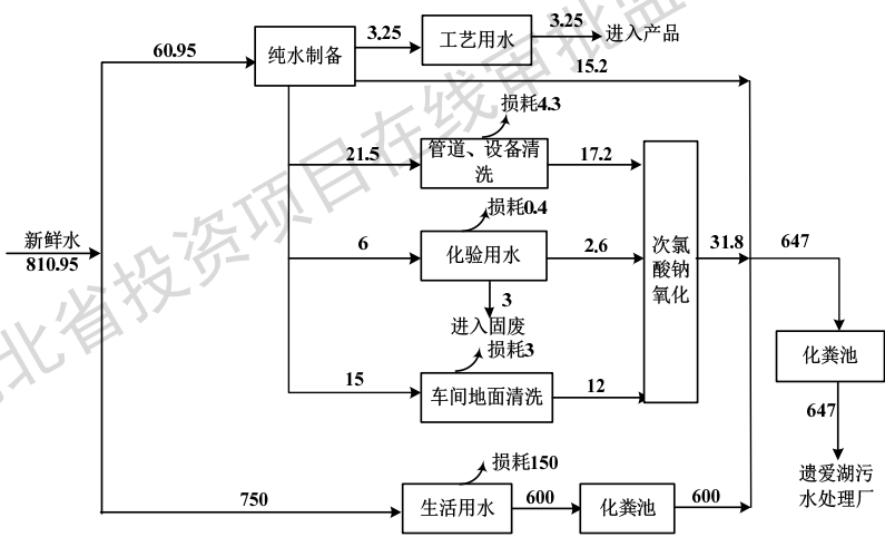
图 2-1 项目全厂水平衡图（单位：m 3 /a）
