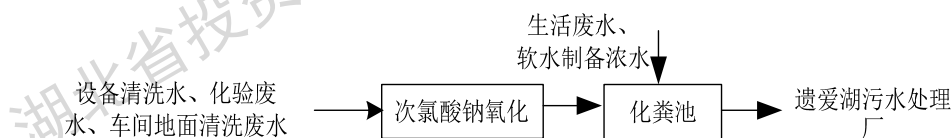
图 4-3 项目污水处理流程图
